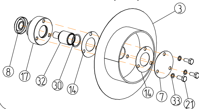
Диск маркёра
