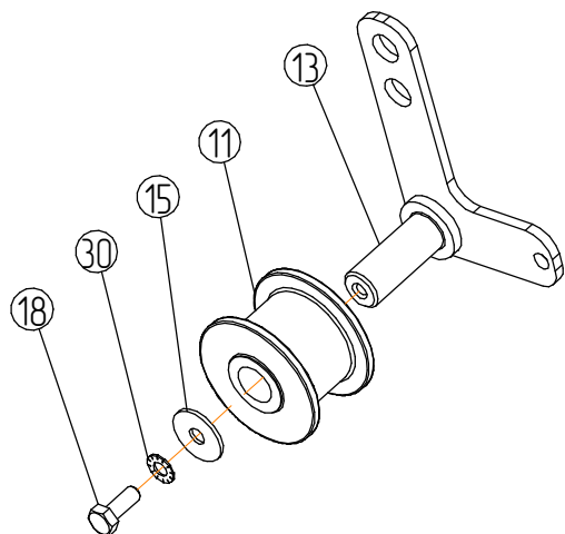
Натяжитель угловой
