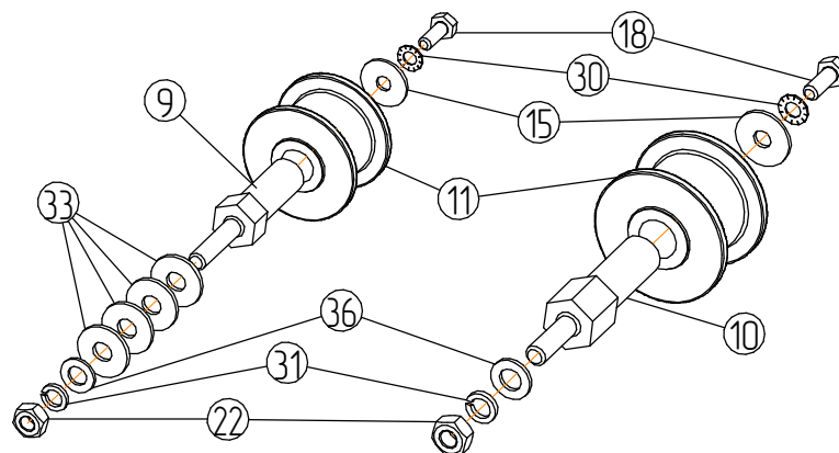
Осевой натяжек
