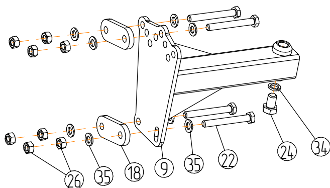
Кронштейн диска
