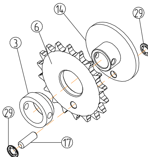
Муфта предохранительная
